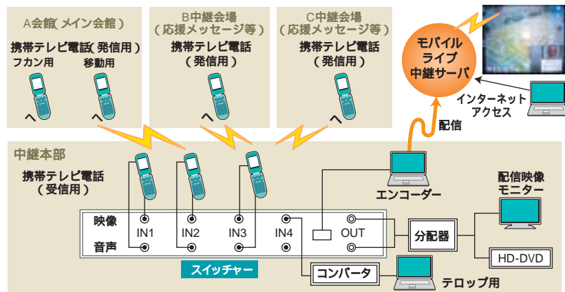
「モバチュウ」基本システム構成図
